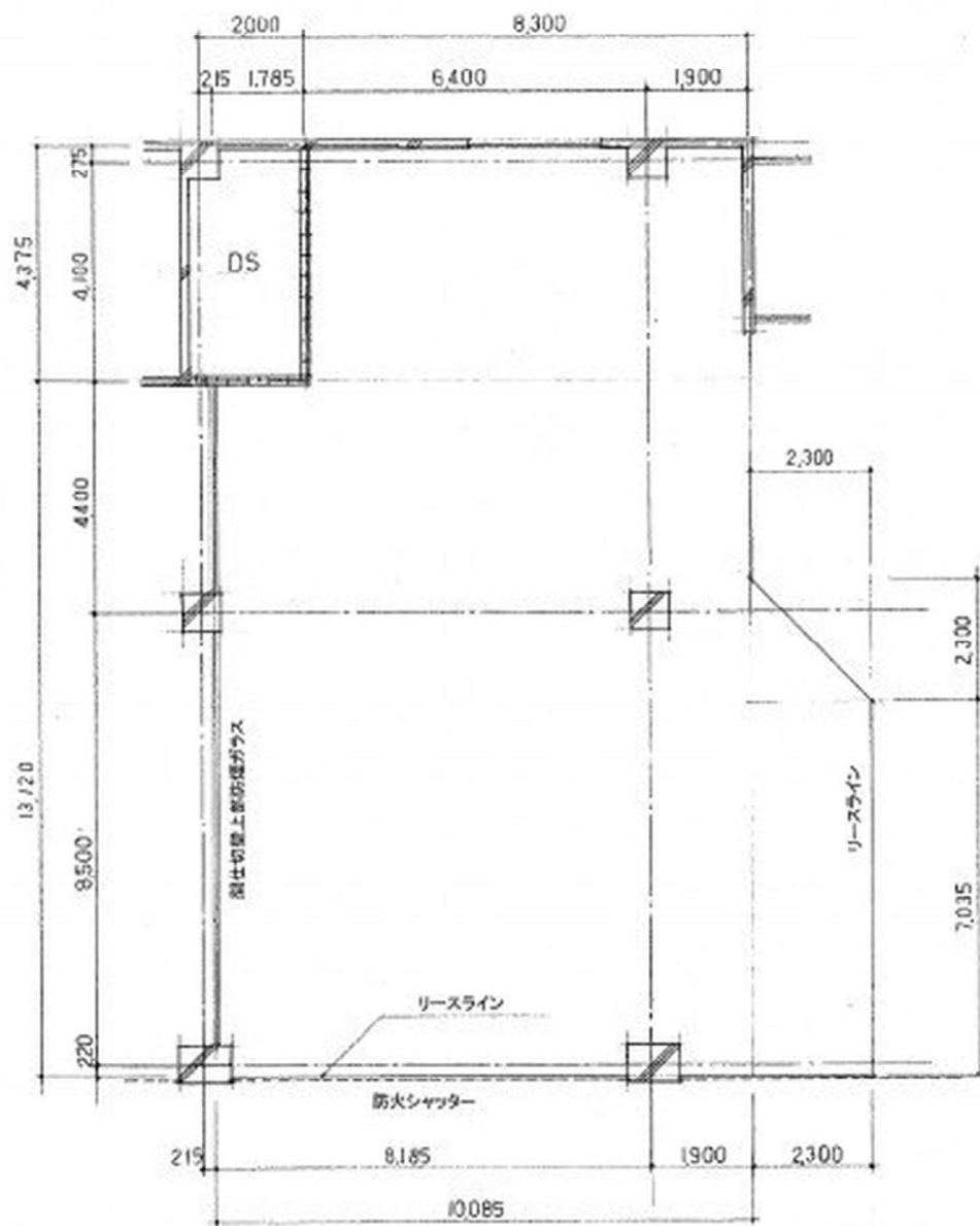
平面图 S:1/100
